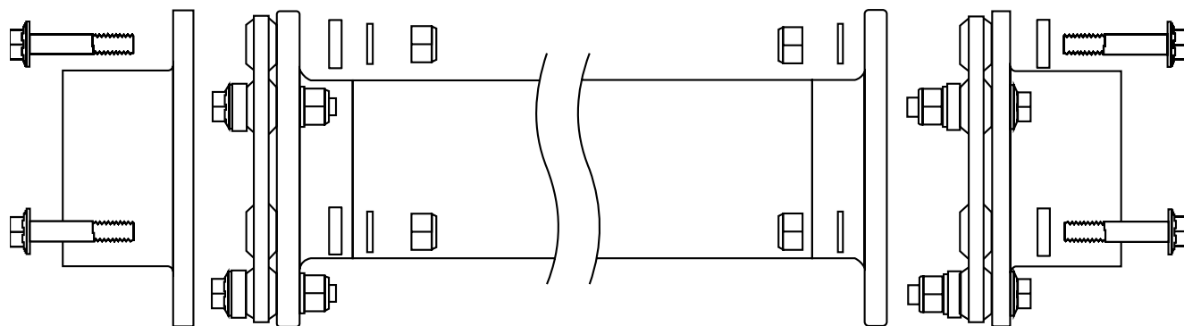
Acoplamento de compósito Addax
